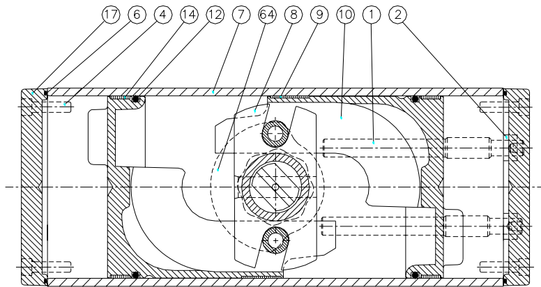
Bild 1 RC265-DA von oben
